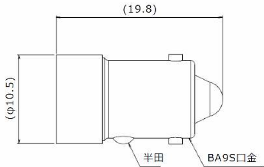
【外形図】
