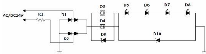
【回路図】
