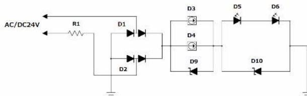
【回路図】
